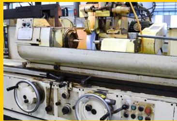
เครื่องเจียรกลม Cylindrical Grinder
